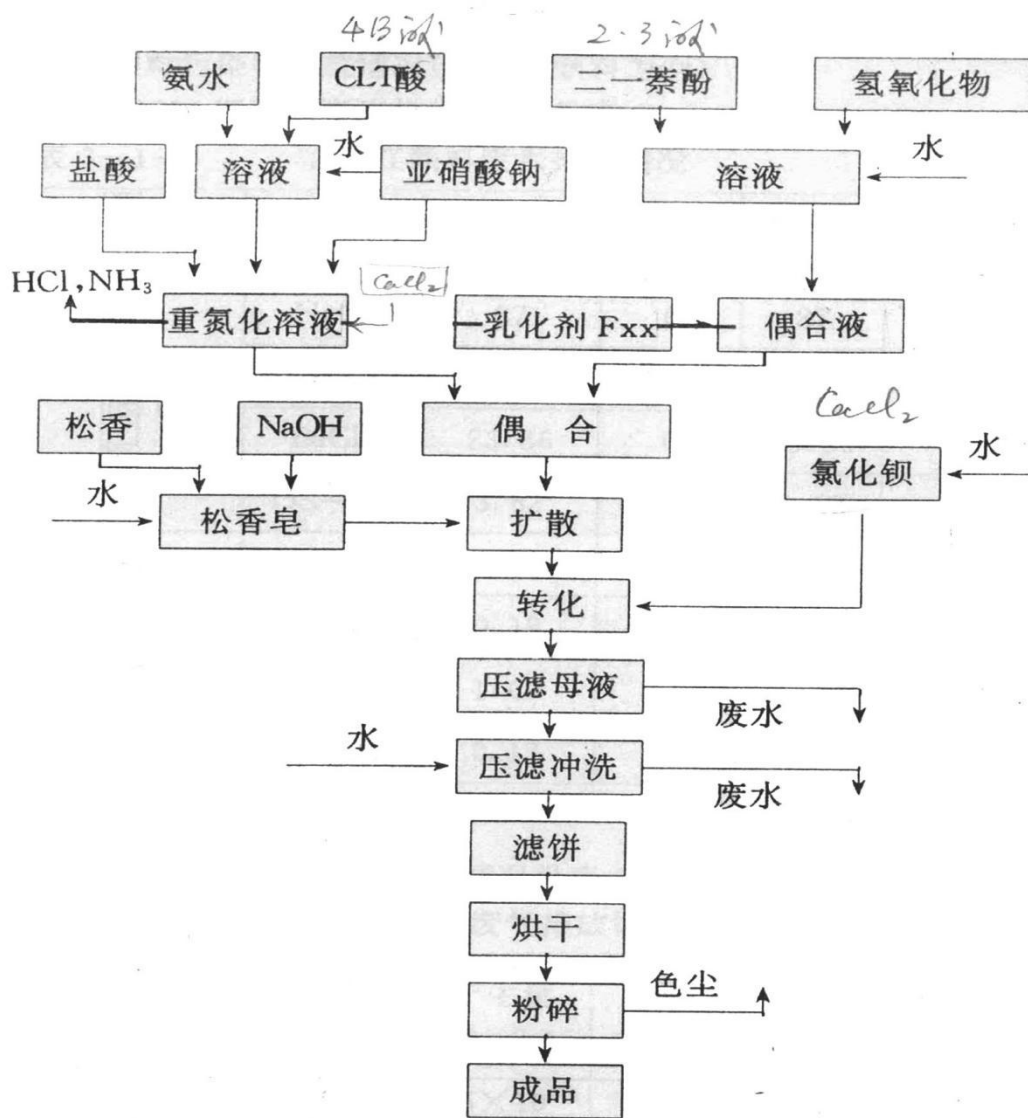
图 2-1-4 红颜料生产工艺流程图
