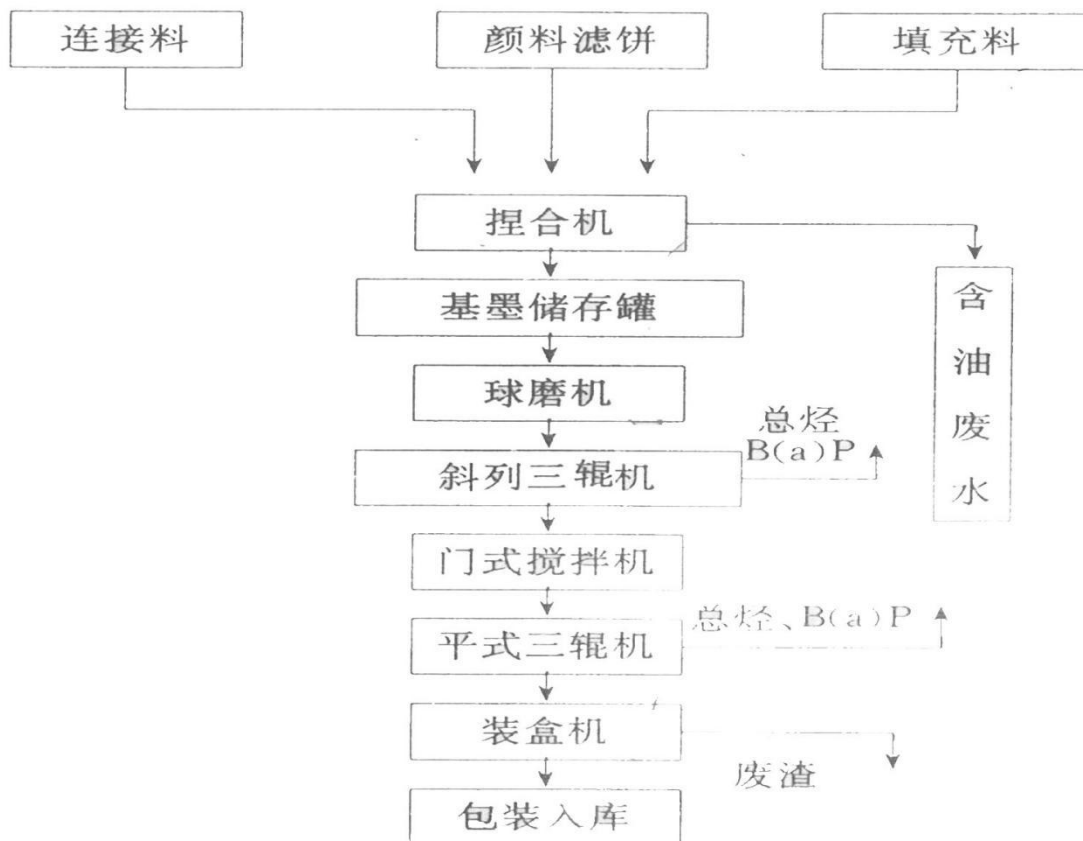
图 2-1-1 油墨生产工艺及污染流程
