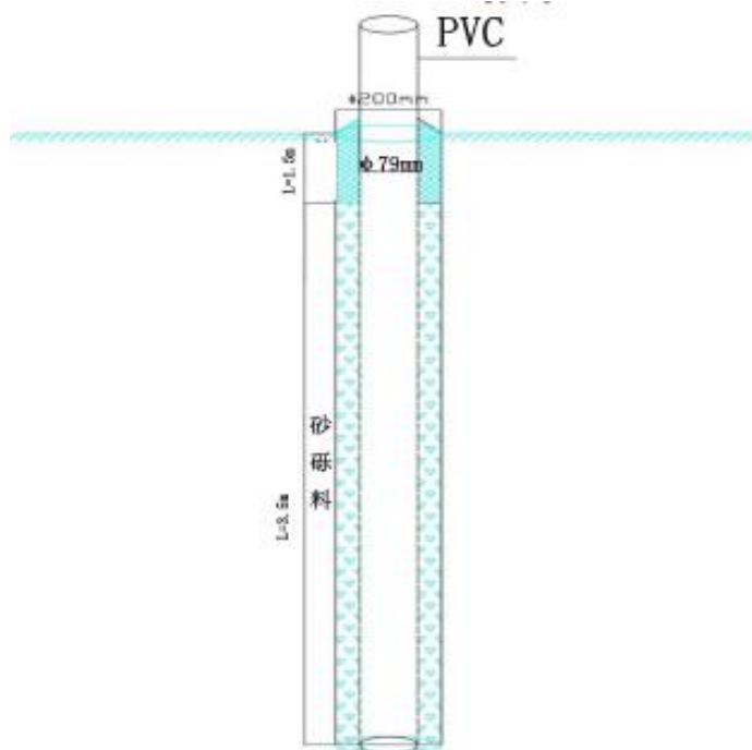
图 2-3-2 地下水监测井结构图
