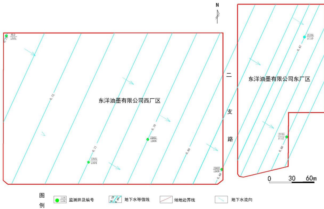
图 2-3-4 厂区地下潜水流场图
