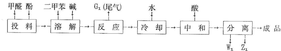
图 2-1-5 油脂基本生产工艺流程图
