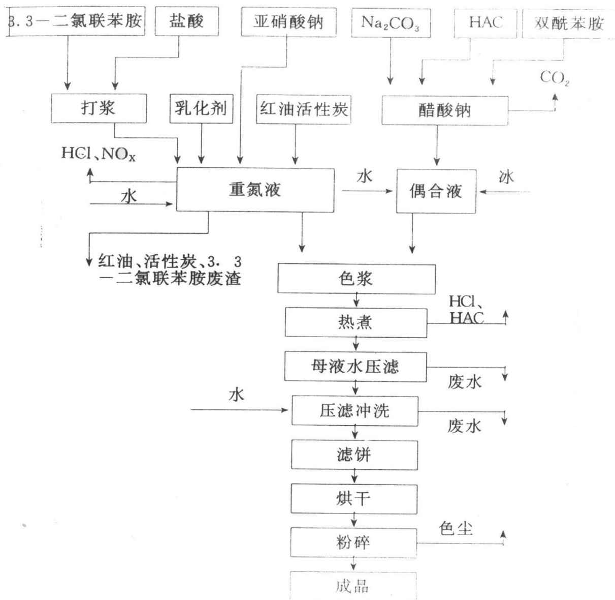
图 2-1-3 黄颜料生产工艺流程图
