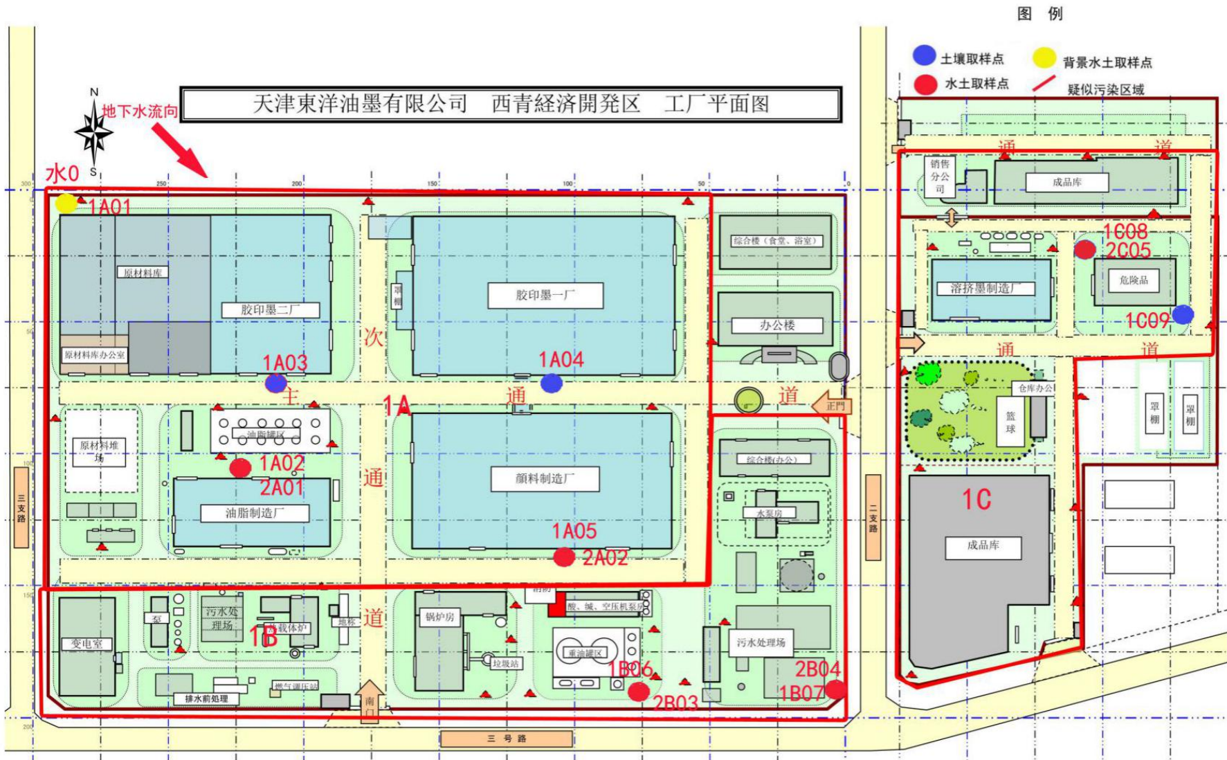
图 3-2-1 监测井及土壤采样布点图
